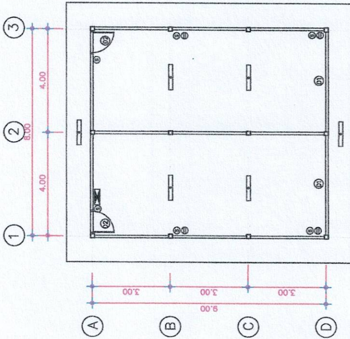
แปลนระบบไฟฟ้าชั้นล่าง มาตราส่วน 1:100
